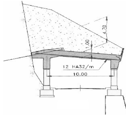
Fig. 1 : Galerie de protection routière conventionnelle
