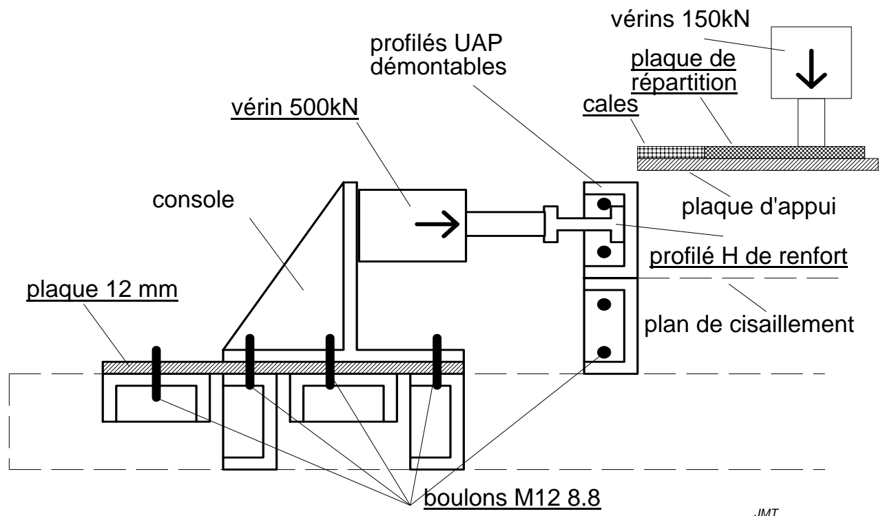
Figure 3 : Boîtier de cisaillement 1000 x 1000 mm - Modifications apportées au bâti
