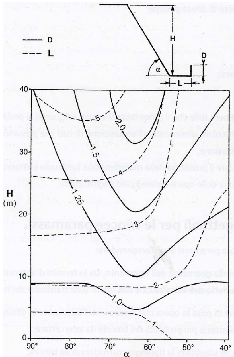
Abaque pour le dimensionnement de la fosse de réception (Whiteside, 1986).
